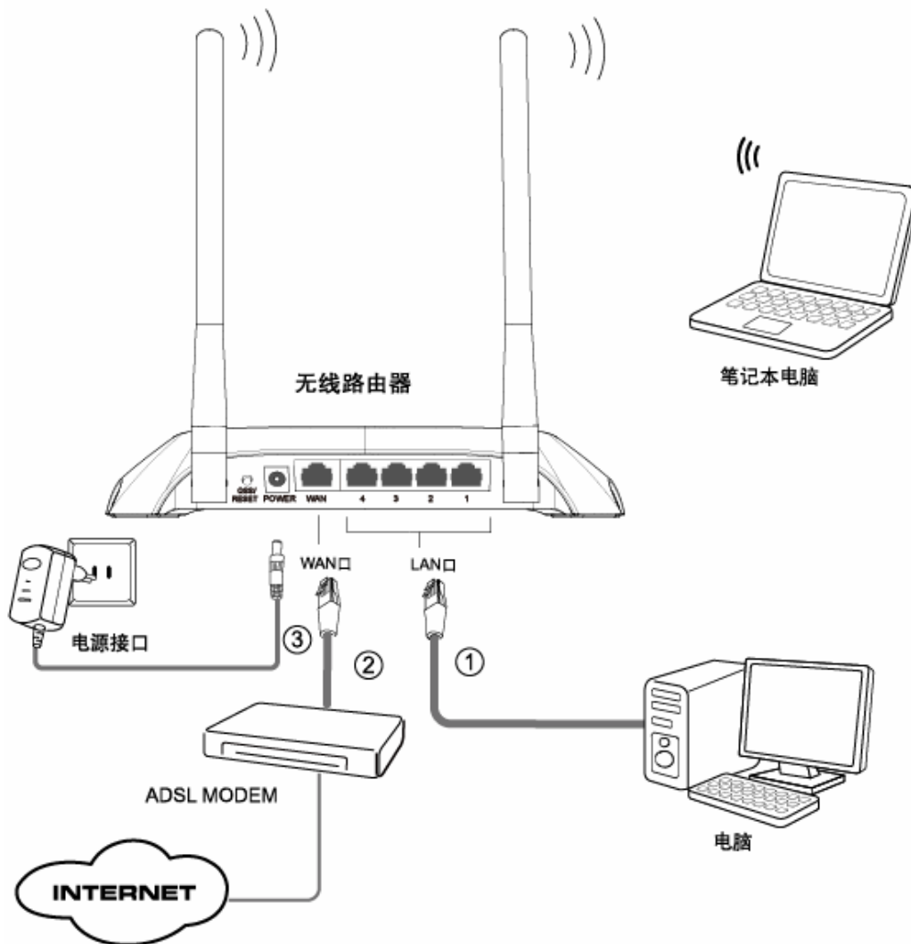
图 4-1 TL-WR841N 硬件安装示意图
